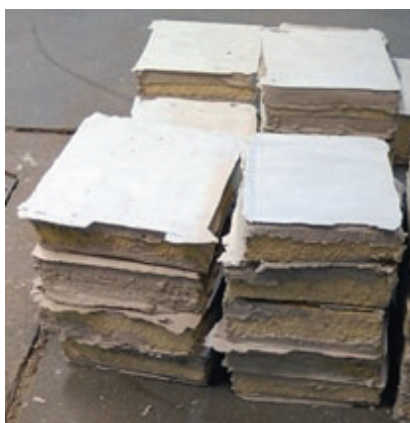
Fot. 2. Próbkę przygotowane do badań, wyrównane warstwą gipsu budowlanego Photo 2. Samples prepared for testing, leveled with a layer of construction gypsum
