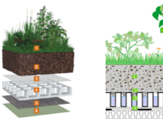
Rysunek 1: Dwa systemy Bauder i Optigrün - porównanie dachu intensywnego [4 i 5]
